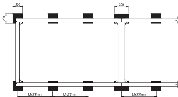
Рис.13 Местные подпорки рам блоков агрегатов
