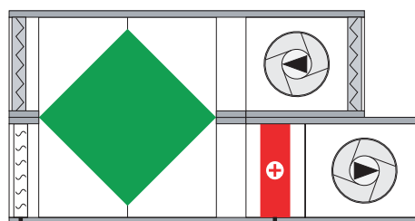
Агрегат с перекрестно-точным теплообменником
