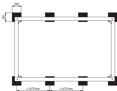
Рис.13 Местные подпорки рам блоков агрегатов
