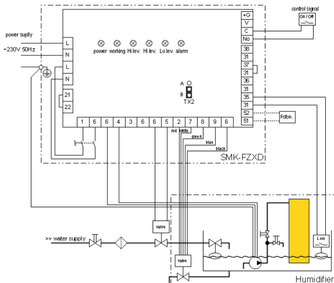
Рис.22.b. Принципиальная схема электрического подключения увлажнителя оборотного водоснабжения. Электрические подключения должны быть выполнены в соответствии со схемами на рис. 22.a и 22.b.
