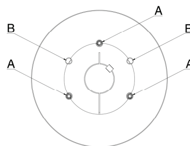
Рис. 33 Шкив с втулками № от 3535 до 5050
